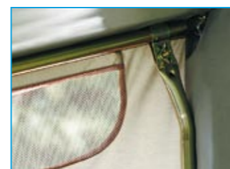
Spezielle Andruckstangen mit angenähten Schaumstoffwülsten sorgen für optimale Abdichtung.
